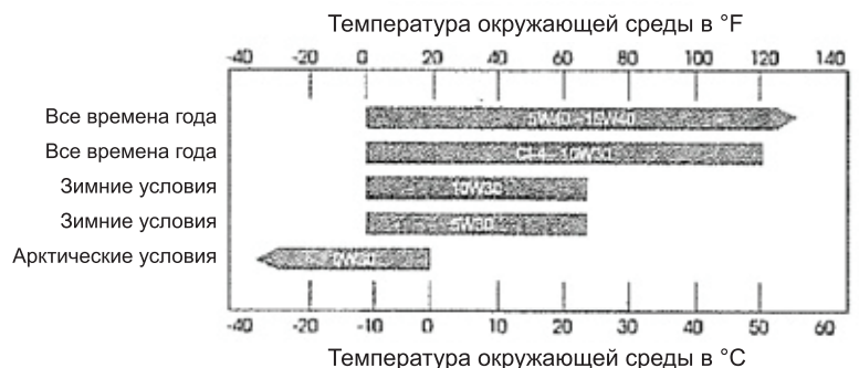
Рисунок: 8.1. Рекомендуемая вязкость/сорта масла в зависимости от температур окружающей среды
