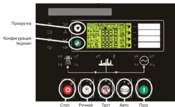
Рис 15.2. Контроллер DSE5220
